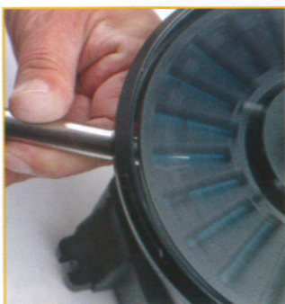
Da die zu schleifende Fläche gut zu sehen ist, können auch gerundete Schneiden risikolos frei Hand geschliffen werden
