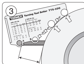
Universalstütze einstellen. Benutzen Sie Loch A oder Loch B.
