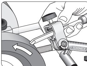
Ziehen Sie die Schneide durch ein Hin- und Herschwenken des Werkzeugs ab. Jetzt haben Sie eine besonders feine Schleiffase.
