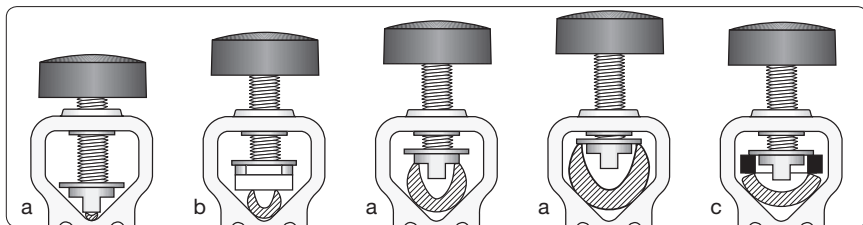
Die spezialkonstruierte Druckplatte passt für Röhren aller Grössen und richtet das Werkzeug so auf, dass es jedes Mal in exakt der gleichen Lage montiert wird. Die Druckplatte kann längs (a) oder quer (b) zum Werkzeug gerichtet werden. Für breite Schalendrehröhren wird eine Scheibe benutzt, die auf die Druckplatte passt (c).
