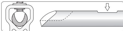
Beim Schleifen eines grossen Drehrohres mit einer kurzen Flute wird die Druckplatte entfernt. Die Oberseite mit einer Feile planen, damit das Schleifen exakt wiederholt werden kann.
