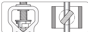
Die Druckplatte funktioniert auch, wenn sie schräg gerichtet ist. (Schnitt von oben gesehen.)
