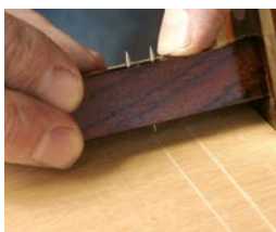
64 Streichmaße
