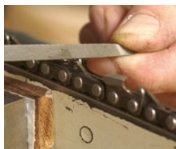
208 Kettensägen
